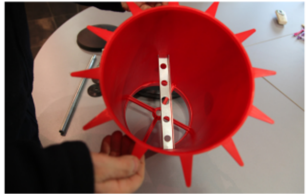
2. Mettre l'entraxe métallique dans le cône
